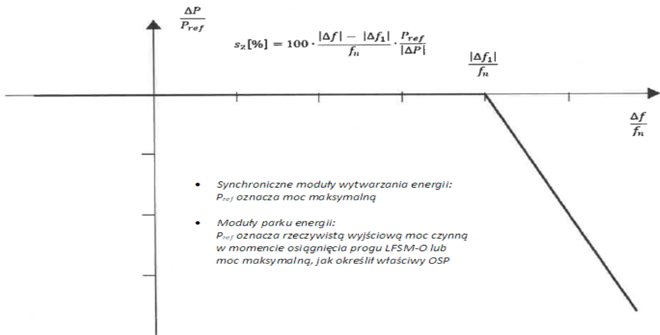
Rys. 1. Zdolność modułów wytwarzania energii do odpowiedzi częstotliwościowej mocy czynnej w trybie LFSM-O
